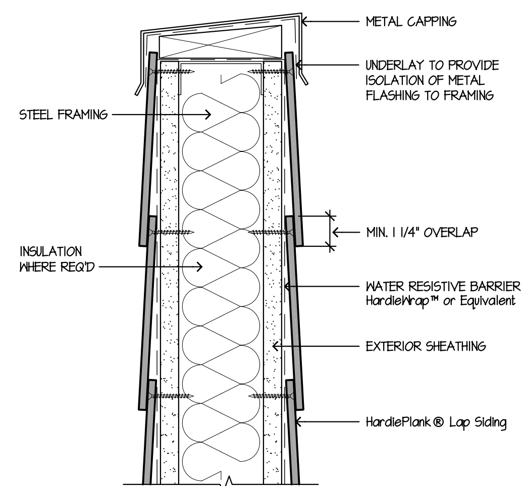
9 PARAPET SCALE: 3/8"=1'-0"
